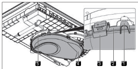
Fig. 9.3 Carcasa de conducción del aire
