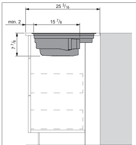
Fig. 11.15 Dimensions de montage pour le dispositif aspirant, profondeur du plan de travail : 25 \frac{3}{16} " [64 cm]
