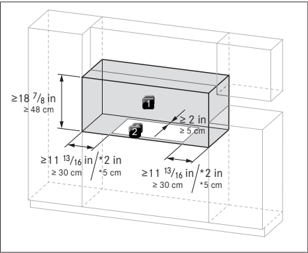
Fig. 11.3 Espacio necesario
