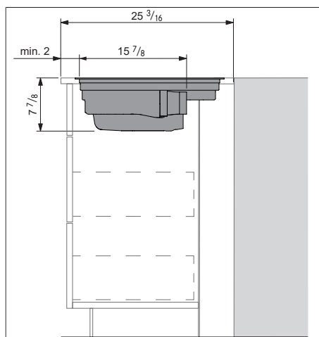
Fig. 11.15 Medidas de instalación para extracción al exterior, profundidad de encimera 25 \frac{3}{16} " [64 cm]
