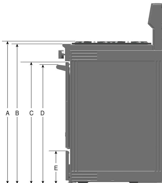
VUE LATÉRALE
