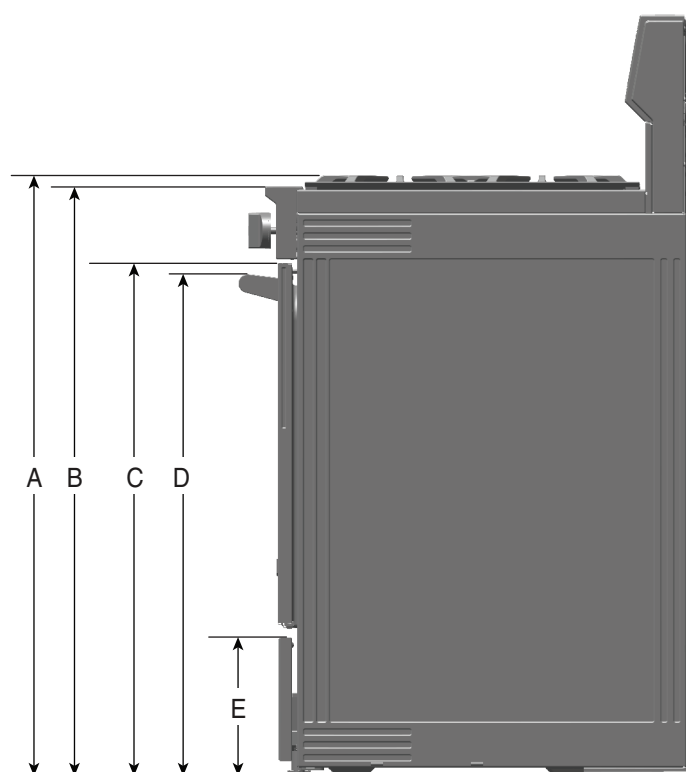
VISTA LATERAL
