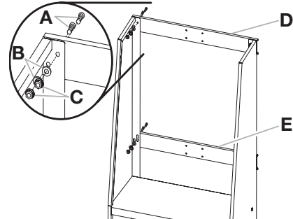
A. Pernos de cabeza redonda (F7) B. Arandela (F8)
