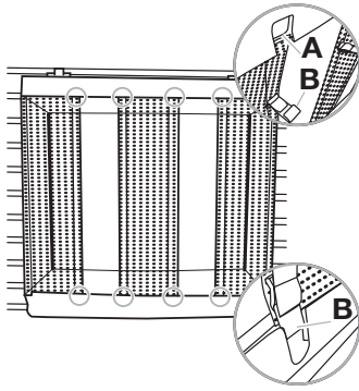
A. Cadre supérieur B. Crochet
