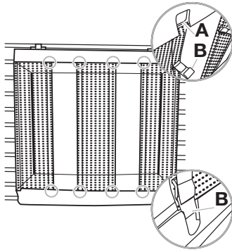
A. Marco superior B. Gancho
