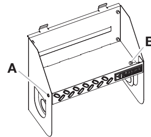
A. Tornillo Phillips (F3b)
