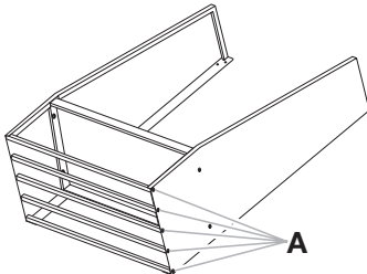
A. Perno de cabeza hexagonal de 5/16" (7,93 mm) (F1)
