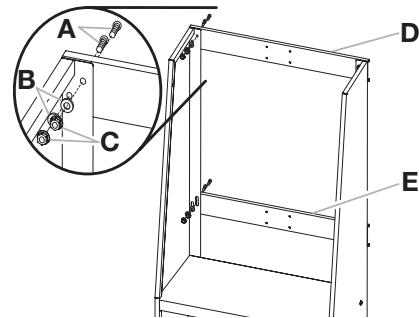
A. Boulon de carrosserie (F7) B. Rondelle (F8) C. Écrous à embase (F2) D. Traverse de fixation supérieure E. Traverse de fixation inférieure
