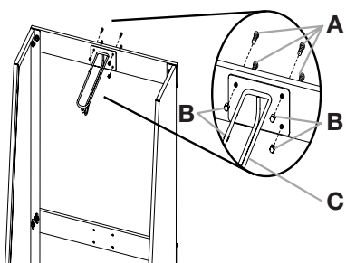
A. Vis à tête cruciforme (F3b) B. Écrous borgnes (F10)
