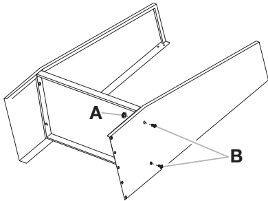
A. Écrou à embase de 5/16 po (7,93 mm) (F2) B. Boulon à tête hexagonale de 5/16 po (7,93 mm) (F1)
