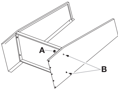
A. Tuerca de brida de 5/16" (7,93 mm) (F2) B. Perno de cabeza hexagonal de 5/16" (7,93 mm) (F1)
