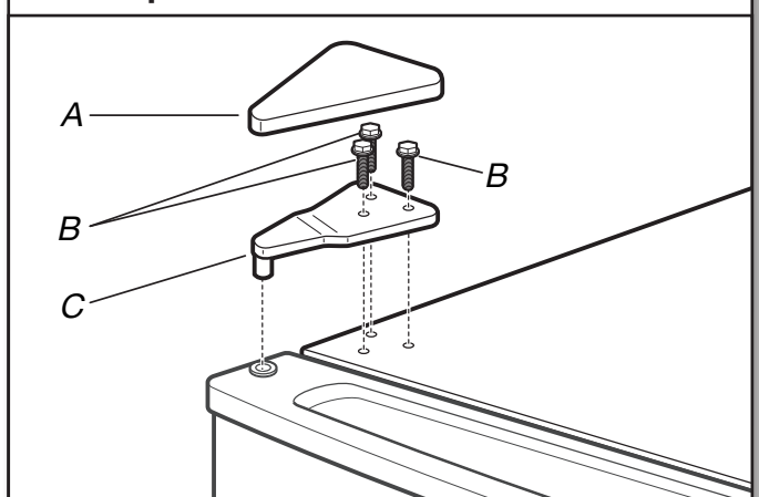
A. Couvercle de charnière supérieure B. Vis de charnière à tête hexagonale de 5/16 po C. Charnière supérieure
