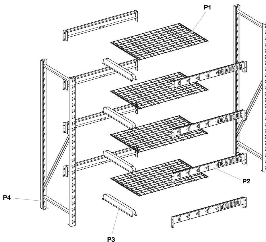
Étagère de 48 po (122 cm) de large
