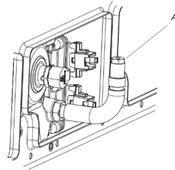
A. Injecteur
