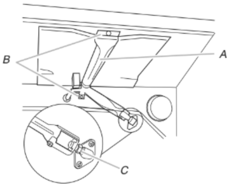
A. Brûleur du grill B. Vis C. Injecteur
