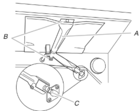
A. Brûleur du gril B. Vis C. Injecteur
