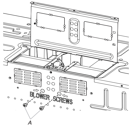
A. Tornillos del soplador (en orificios embutidos)
