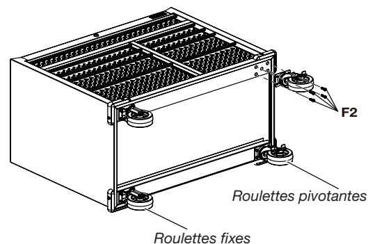
F2. Boulons à tête hexagonale (M8 - 1,25 x 25)
