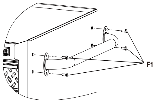
F1. Boulons à tête hexagonale (M6 - 1,00 x 15)
