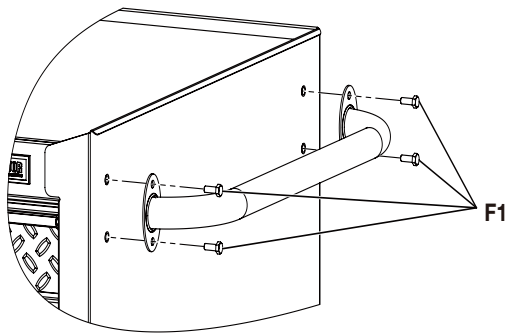
F1. Pernos de cabeza hexagonal (M6 - 1,00 x 15)
