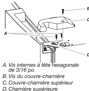
Charnière supérieure droite
