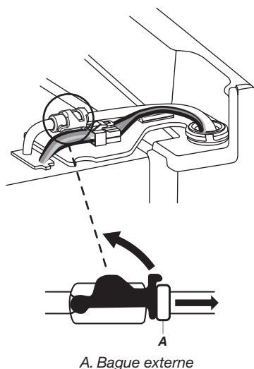
Style 2 – Raccord de tuyau du distributeur d'eau
