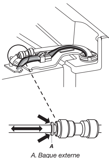
Style 1 – Raccord de tuyau du distributeur d'eau
