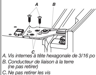
Charnière supérieure gauche
