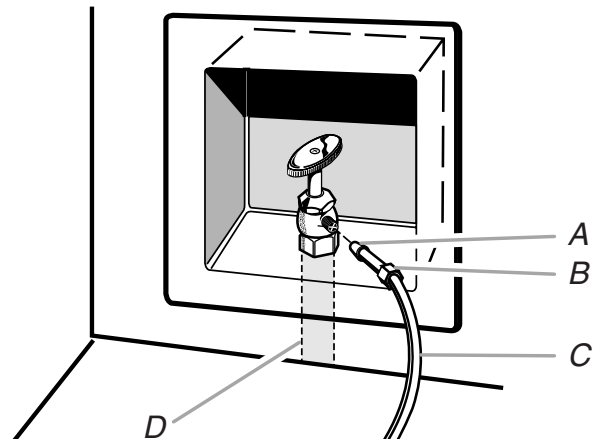
A. Bague C. Canalisation en cuivre (jusqu'au réfrigérateur) B. Écrou D. Canalisation d'alimentation du domicile (1/2 po (12,7 mm) minimum)
