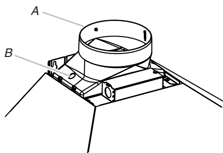
A. Raccord de transition B. Vis 3,5 mm x 9,5 mm
