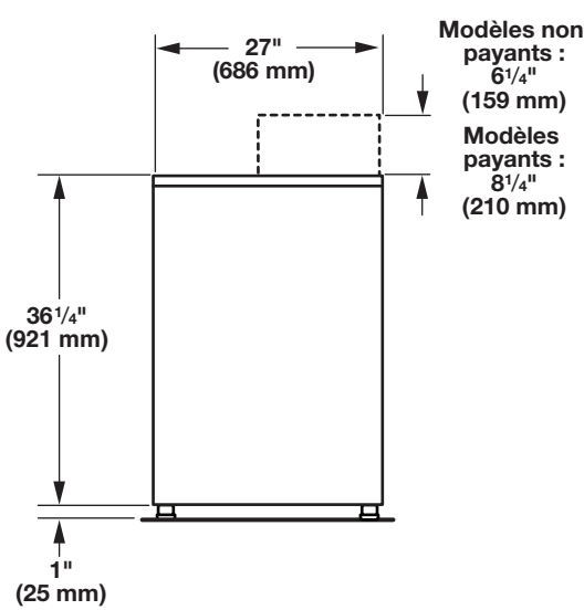
Vue latérale
