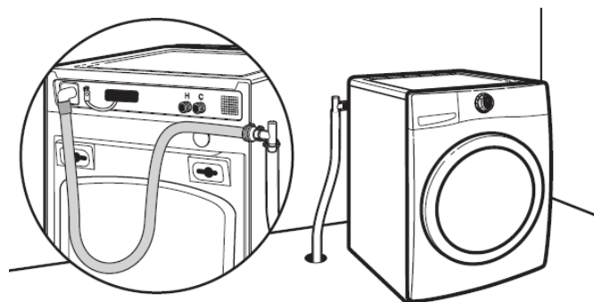
Figura 5 – Sistema de desagüe de piso – Carga frontal
