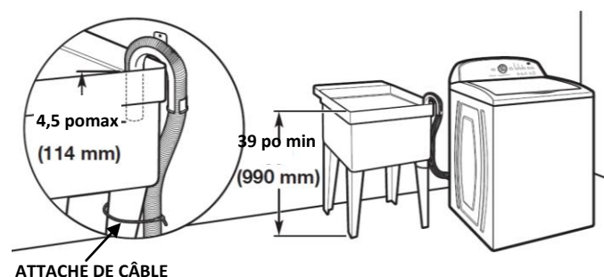
Figure 3 – Évacuation via un bac de buanderie
