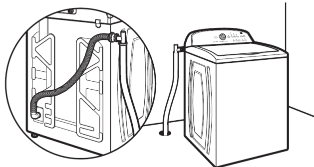
Figure 4 – Évacuation par le plancher – Chargement par le sommet
