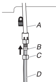
A. Canalisation d'eau en plastique B. Manchon
