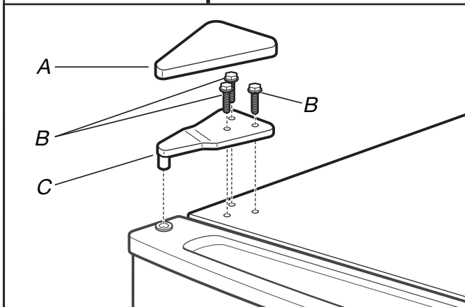
A. Couvercle de charnière supérieure
