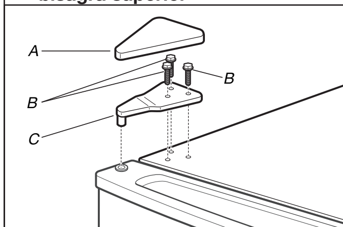
A. Cubierta de bisagra superior
