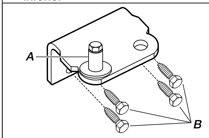
A. Pasador de la bisagra inferior
