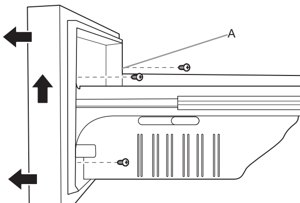
A. Ranuras del soporte de la guía del cajón
