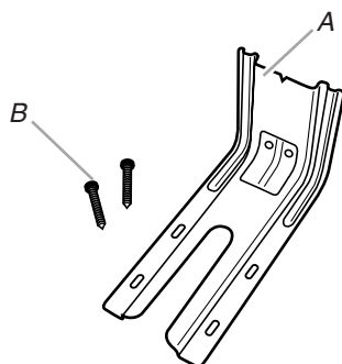
A. Soporte antivuelco B. Tornillos n° 12 x 1 5/8" (2)
