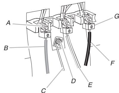
A. Tuerca hexagonal 10-32 B. Línea 2 (roja) C. Hilo desnudo de conexión a tierra (verde) D. Tornillo de puesta a tierra E. Hilo neutro (blanco) F. Línea 1 (negro) G. Lengüeta de terminal
