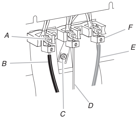
A. Tuerca hexagonal 10-32 B. Línea 2 (roja) C. Tornillo de puesta a tierra D. Hilo desnudo de conexión a tierra (verde) E. Línea 1 (negra) F. Lengüeta de terminal
