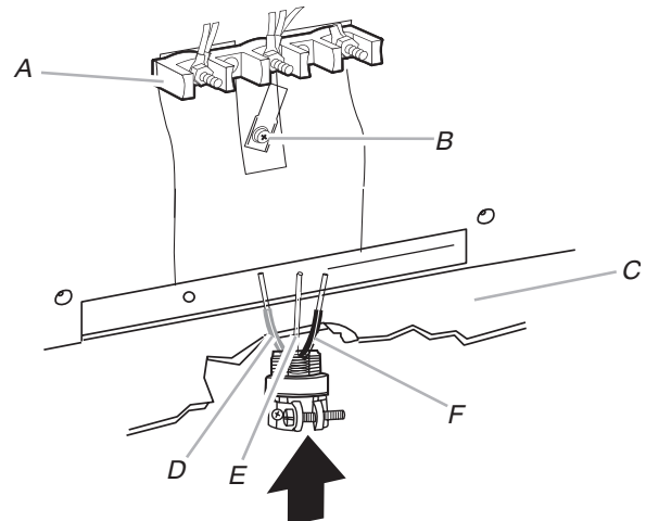
A. Bloque de terminales B. Tornillo de puesta a tierra C. Placa de cable/conducto D. Hilo de línea 2 (rojo) E. Hilo desnudo de conexión a tierra (verde) F. Hilo de línea 1 (negro)
