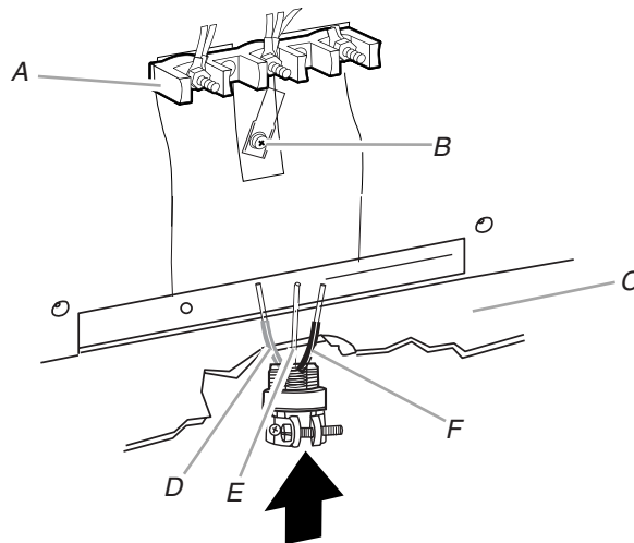
A. Bornier B. Vis de liaison à la terre C. Plaque de cordon/conduit D. Conducteur de ligne 2 (rouge) E. Fil de mise à la terre nu (vert) F. Conducteur de ligne 1 (noir)
