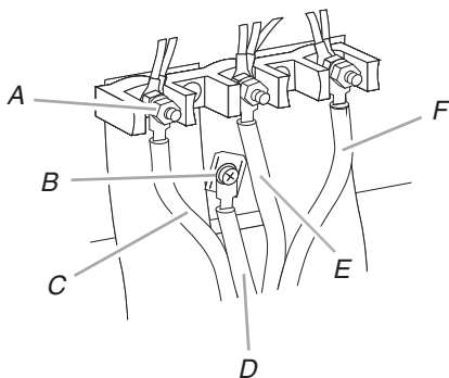
A. Tuerca hexagonal 10-32 D. Hilo de conexión a tierra (verde) B. Tornillo de enlace a tierra E. Hilo neutro (blanco) C. Hilo de línea 2 (rojo) F. Hilo de línea 1 (negro)
