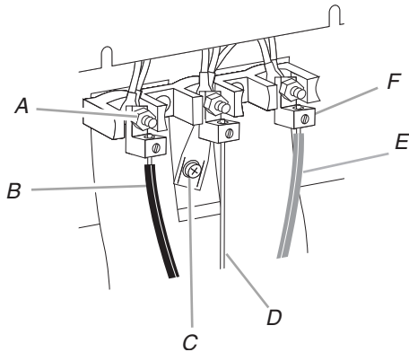
A. Tuerca hexagonal 10-32 B. Hilo de línea 2 (rojo) C. Tornillo de enlace a tierra D. Hilo desnudo de conexión a tierra (verde) E. Hilo de línea 1 (negro) F. Lengüeta de terminal
