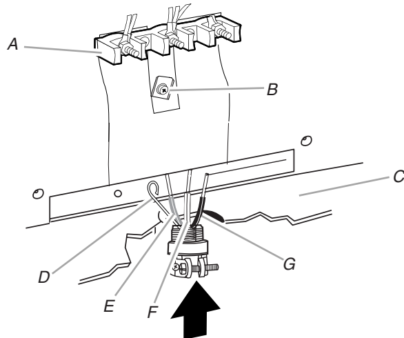
A. Bloque de terminales B. Tornillo de enlace a tierra C. Placa de cable/conducto D. Hilo desnudo de conexión a tierra (verde) E. Hilo de línea 2 (negro) F. Hilo neutro (blanco) G. Hilo de línea 1 (negro)
