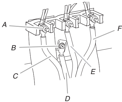
A. Écrou hexagonal 10-32 B. Vis de liaison à la terre C. Conducteur de ligne 2 (rouge) D. Fil de mise à la terre vert E. Conducteur neutre (blanc) F. Conducteur de ligne 1 (noir)
