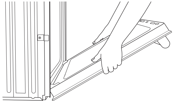
A. Loquet de charnière de la porte du four en position de verrouillage
