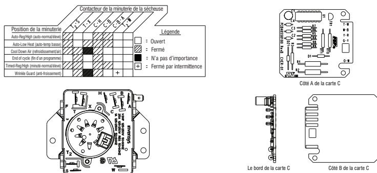
Figure 8 - Schémas de la minuterie et de la carte C, sècheuse électrique de 120V
