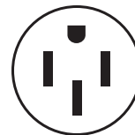
Réceptacle de 4 fils (14-50P)
