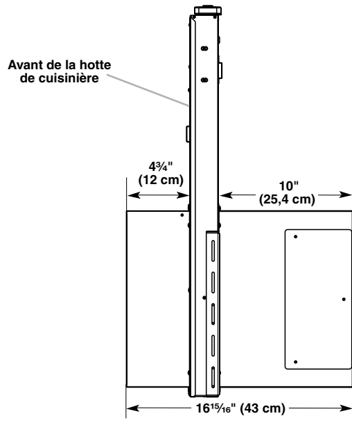
Ventilateur inversé
