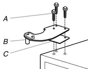
A. Vis de charnière à tête hexagonale de 5/16" B. Axe de charnière supérieure
