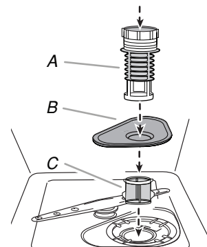
A. Filtre principal B. Filtre métallique C. Tamis fin
