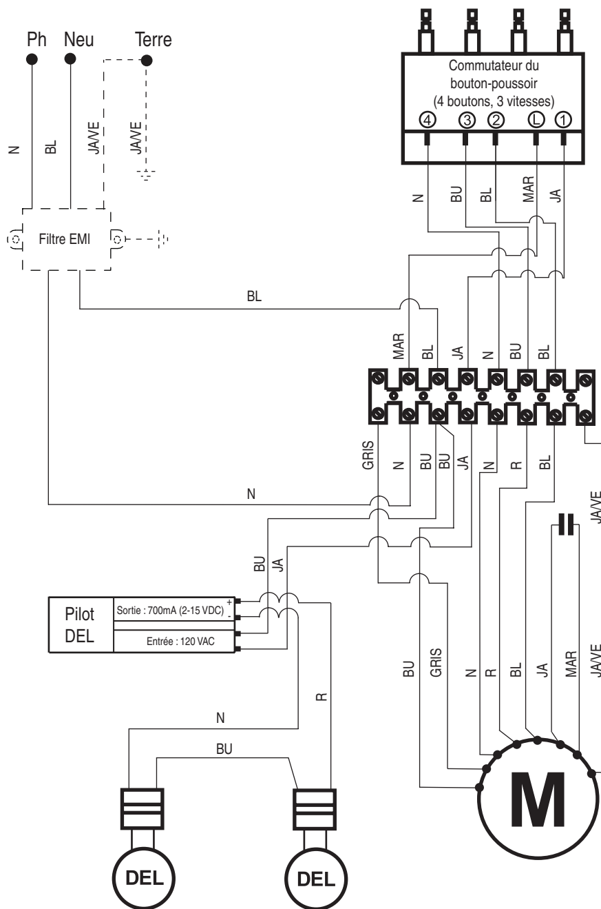
Fonctionnement du commutateur du bouton-poussoir
