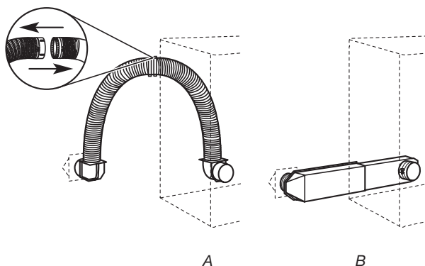
A. Installation au-dessus de la sècheuse (également disponible avec un coude décalé) B. Installation de périscope
