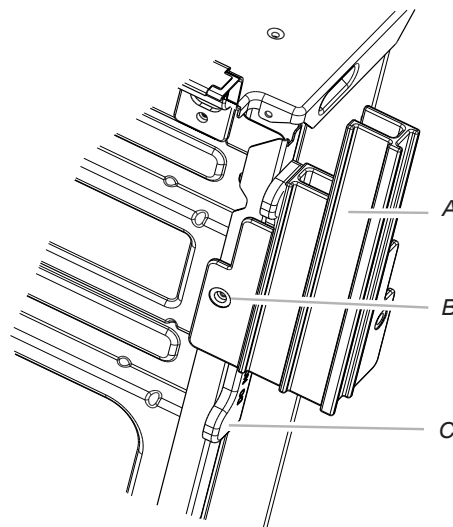
A. Pied avant B. Vis n° 8-18 x \frac{3}{8} " C. Cale d'espacement
