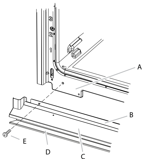
A. Châssis du four D. Garniture de l'évent inférieur B. Support de l'évent E. Vis n° 8-18 x 3/8" C. Évén du four
