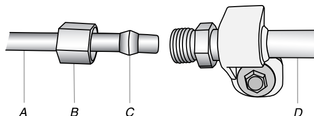
A. Canalisation d'eau du domicile B. Écou (à acheter) C. Virole (à acheter) D. Conduit d'eau vers le réfrigérateur
