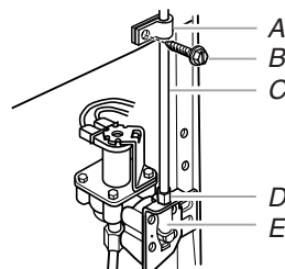
A. Bride du tube B. Vis de bride de tube C. Tube en cuivre D. Écou de compression E. Valve d'entrée d'eau
