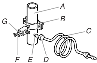
A. Canalisation d'eau froide B. Bride de tuyau C. Tube en cuivre D. Écou de compression E. Bague de compression F. Robinet d'arrêt G. Écou de serrage
