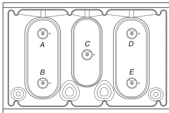
A. Standard burner - LP gas orifice spud number 78
