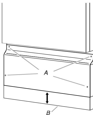
A. 4 trous de vis supérieurs B. Plinthe à 2 pièces
