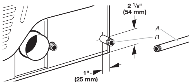
A. Canalisation d'arrivée de gaz NPT de 1/2" B. Tuyau NPT de la sècheuse de 3/8"
