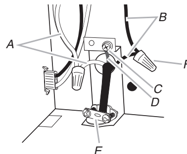
A. Conducteurs blancs B. Conducteurs noirs C. Vis verte de liaison à la terre D. Conducteur de liaison à la terre E. Serre-câble (homologation UL ou CSA) F. Connecteur de fils
