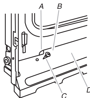
A. Oven frame slot
