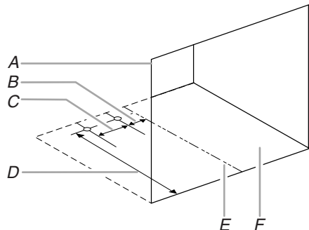
A. Ouverture découpée B. 1\frac{3}{16} " (2,06 cm) C. 3" (7,62 cm) D. 16\frac{3}{4} " (42,55 cm) E. Axe central F. Plancher de la cavité
