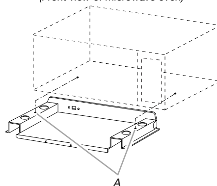
A. ½" screws
