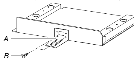
A. Bride du fond B. Vis de 1/2"
