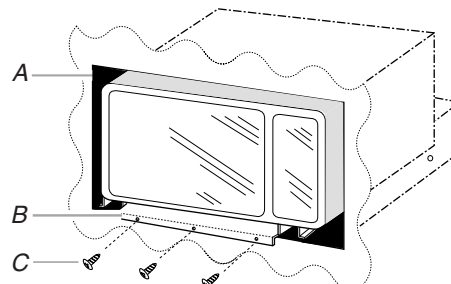
A. Ouverture découpée de la cavité B. Collerette de positionnement C. Vis de \frac{1}{2} "
