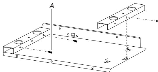
A. ½" screws
