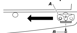
A. Door Stop B. Door Stop Screw
