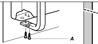
A. Tornillos de cabeza plana para la manija B. Manija del congelador
