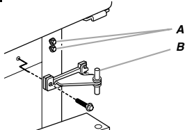
A. Vis de charnière à tête hexagonale de 5/16" B. Charnière centrale
