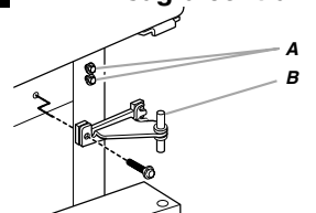
A. Tornillos de cabeza hexagonal para bisagra de 5/16" B. Bisagra central
