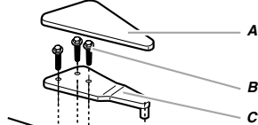
A. Tapa de la bisagra superior B. Tornillos de cabeza hexagonal para bisagra de \frac{5}{16} " C. Bisagra superior
