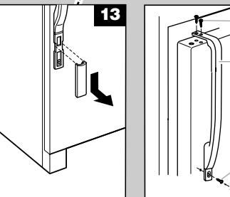
A. Tornillo de cabeza plana para la manija B. Manija del refrigerador C. Tornillo de la manija D. Tapa del tornillo de la manija de la puerta
