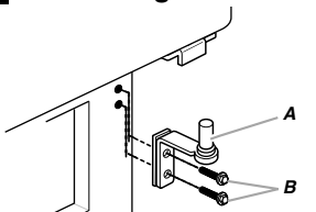
A. Bisagra inferior B. Tornillos de cabeza hexagonal para bisagra de 5/16"
