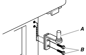
A. Bisagra inferior B. Tornillos de cabeza hexagonal para bisagra de \frac{5}{16} "
