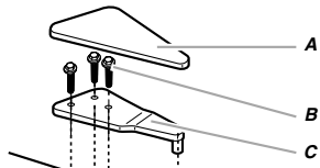
A. Couverture de la charnière supérieure B. Vis de charnière à tête hexagonale de 5/16" C. Charnière supérieure
