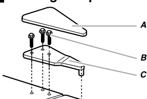
A. Tapa de la bisagra superior B. Tornillos de cabeza hexagonal para bisagra de 5/16" C. Bisagra superior
