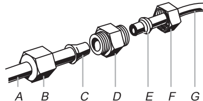
A. Tubería de agua del refrigerador B. Tuerca (provista) C. Bulbo D. Acoplamiento (provisto) E. Fécula (adquirida) F. Tuerca (adquirida) G. Línea de agua de la casa
