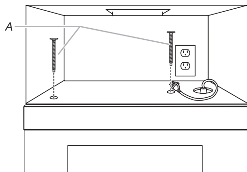
A. Bolts
