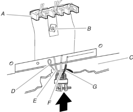
A. Bloque de terminales B. Tornillo de enlace a tierra C. Placa de cable/conducto D. Hilo desnudo de conexión a tierra (verde) E. Hilo de línea 2 (rojo) F. Hilo neutro (blanco) G. Hilo de línea 1 (negro)
