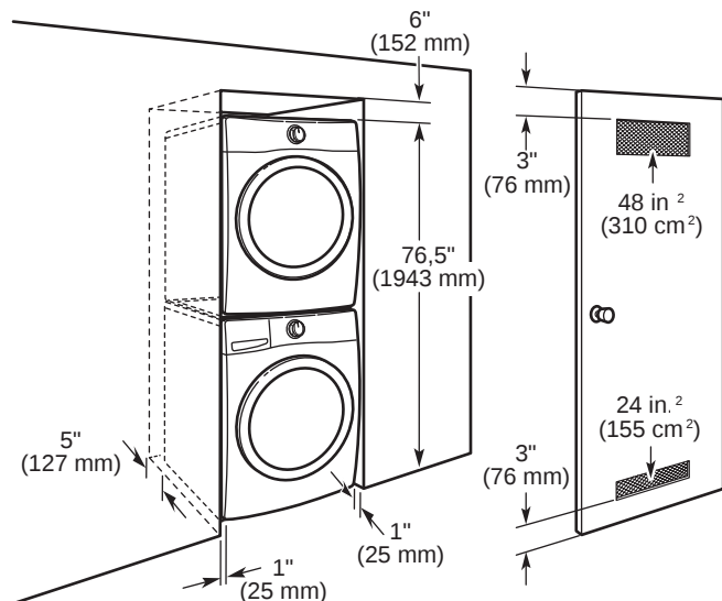
Instalación en zona empotrada o en clóset (lavadora y secadora apiladas):
