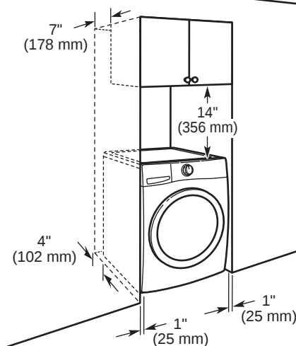
Instalación con armarios a la medida:
