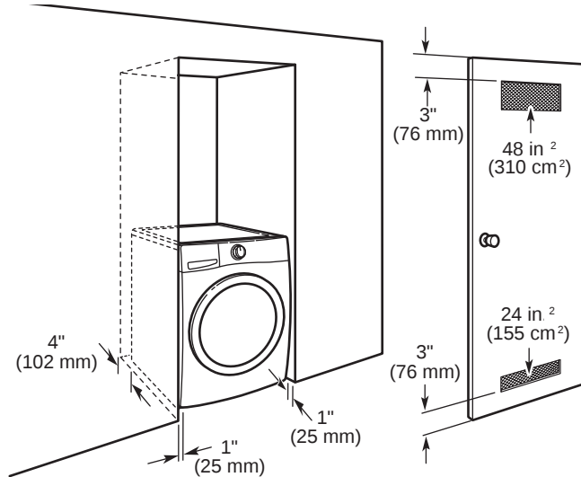
Instalación en zona empotrada o en clóset (sólo lavadora):
