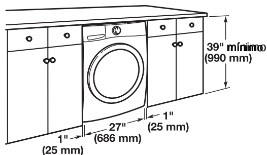
Instalación bajo mostradores a la medida:
