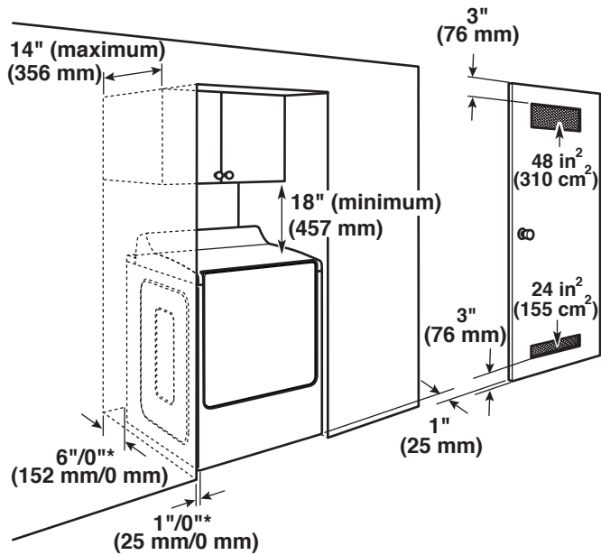
Espacios mínimos/recomendados
