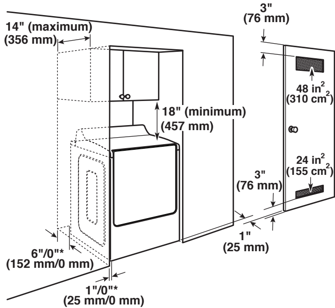
Espacios mínimos/recomendados
