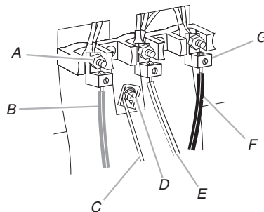
A. Écrou hexagonal 10-32 B. Ligne 2 (rouge) C. Conducteur de mise à la terre nu (vert) D. Vis de liaison à la terre E. Conducteur neutre (blanc) F. Ligne 1 (noir) G. Cosse
