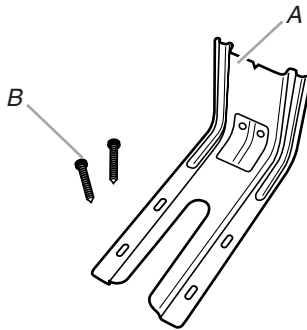
A. Bride antibascullement B. 2 Vis n° 12 x 1 5/8" (4,1 cm)
